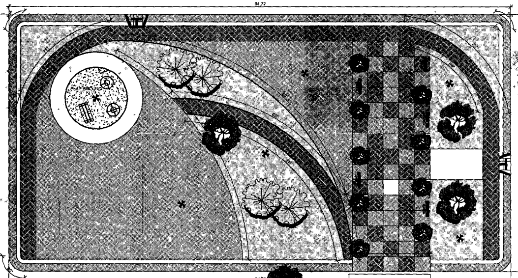
PLANTA BAIXA E PLANTA DE IMPLANTAÇÃO
